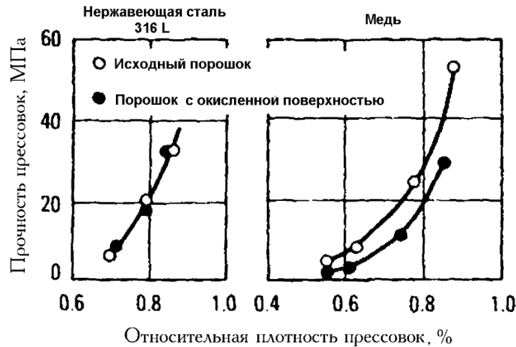
Рис. 5. Влияние поверхностных оксидных пленок на прочность прессовок из порошков меди и нержавеющей стали 316L [19]
